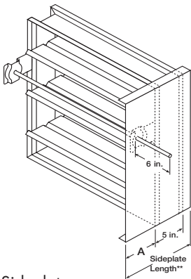
Sideplate
