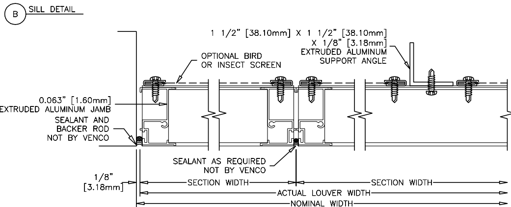
C JAMB DETAIL
